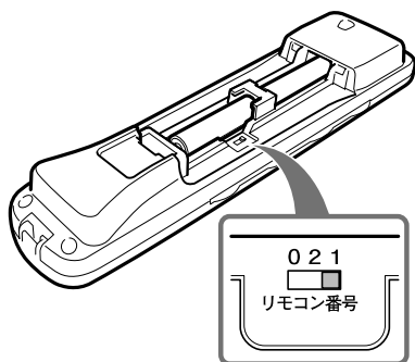
▲リモコン番号 切換スイッチ
